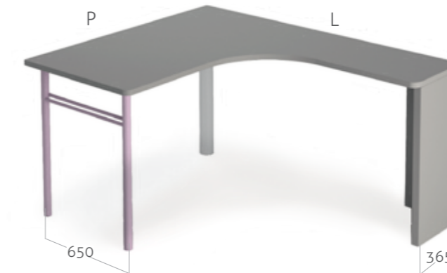
TIPOLOGIA "61.62.63" L.1200-1350-1500-1650-1800 P.1050-1200-1350
