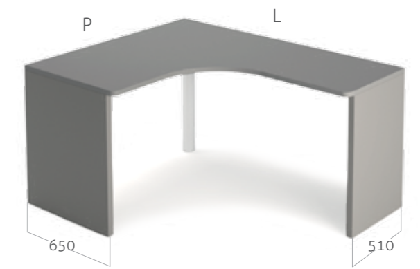
TIPOLOGIA "67.68.69" L.1200-1350-1500-1650-1800 P.1050-1200-1350
